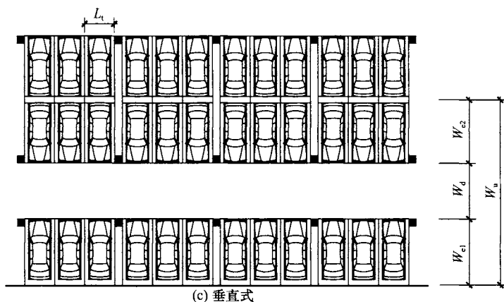
图 4.3.3 停车方式 (二)
