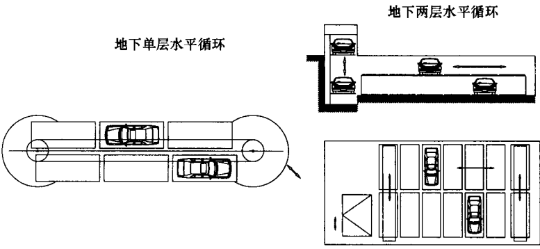
图 3 水平循环类停车设备示意图
