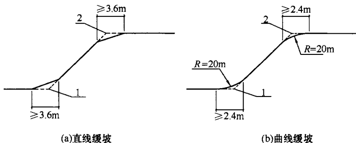
图 4.2.10 缓坡
