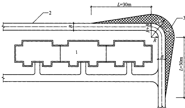
图 10 场地内消防车道的弯道设计示意图
